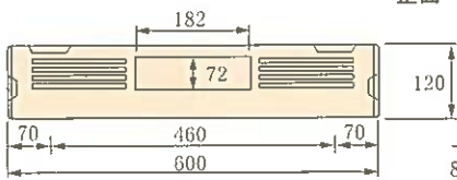
NSP-100A 参考重量 18kg
