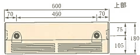
NSP-120B 参考重量 25kg
