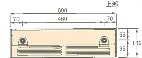
NSP-100B 参考重量 18kg
