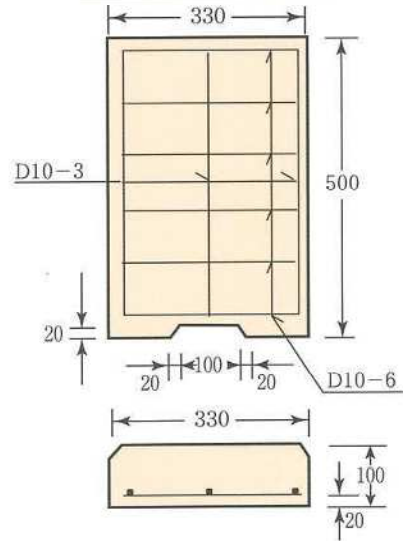
PC6型-240
